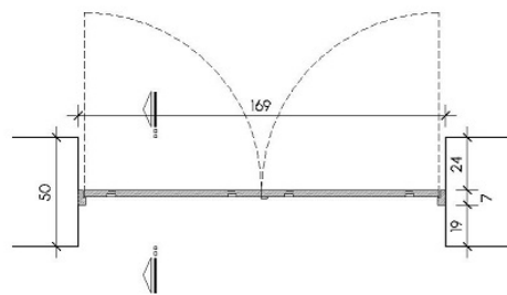
Planta Baixa
