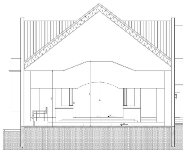
Corte BB
