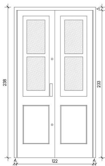
Vista Interna
