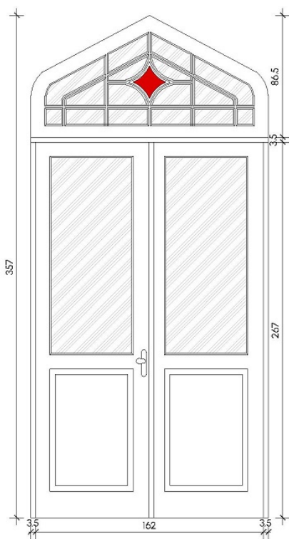
Vista Interna
