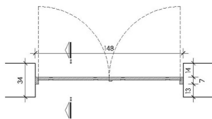
Planta Baixa
