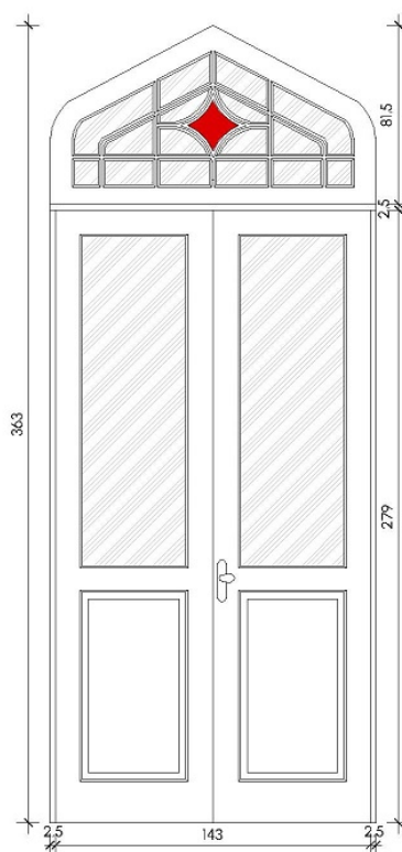
Vista Externa
