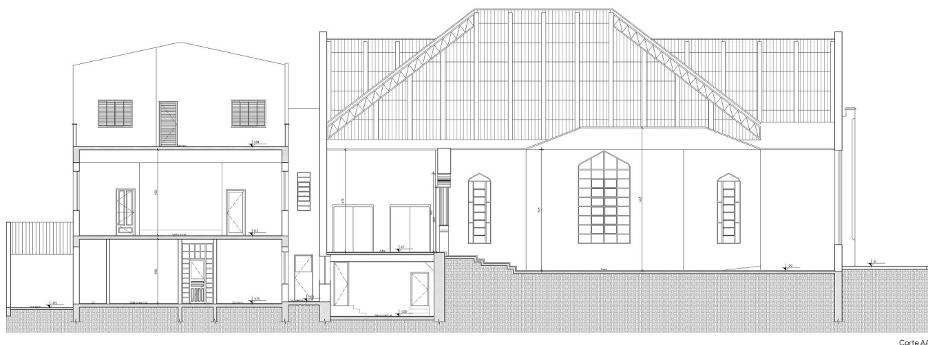
Corte AA
