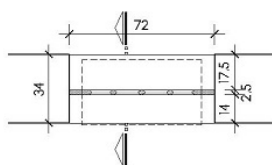
Planta Baixa
