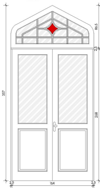
Vista Externa
