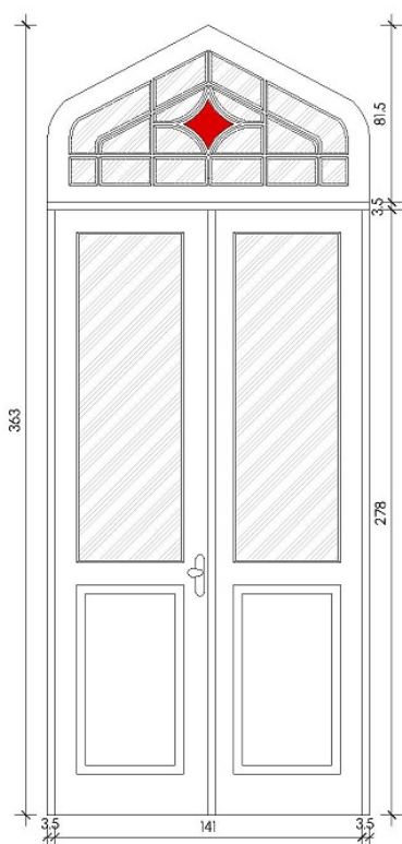
Vista Interna
