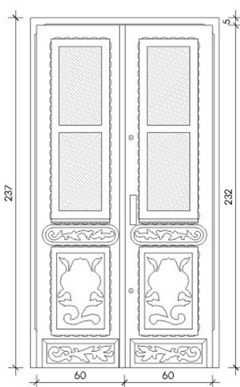
Vista Externa
