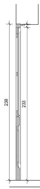
Corte
